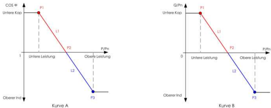
Abbildung 8-3 Q(P)-Kurve
